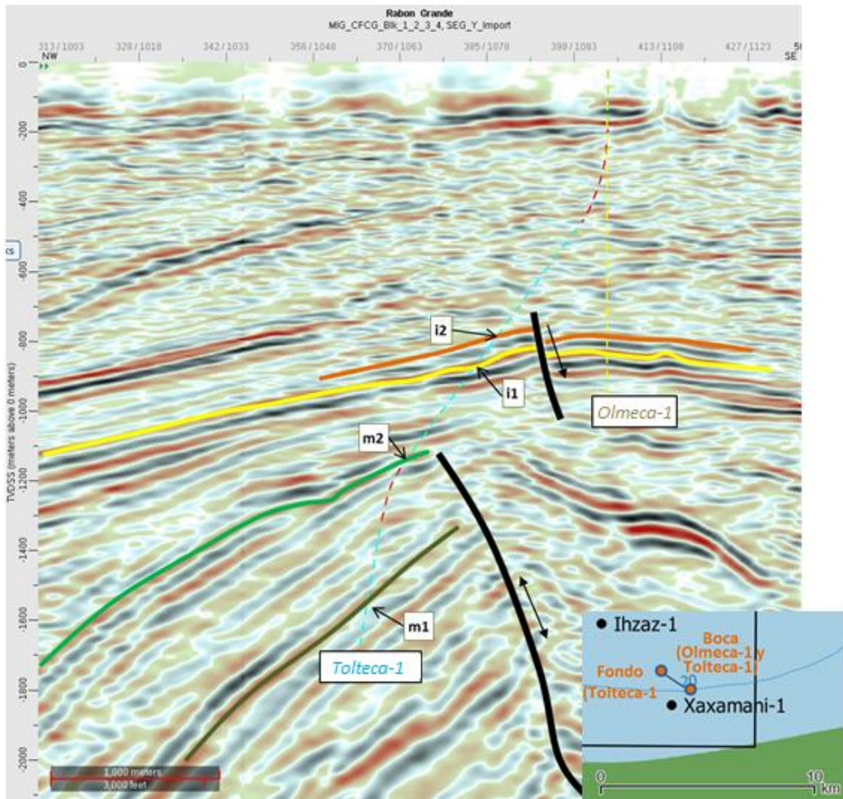
Figura 3. Sección sísmica
